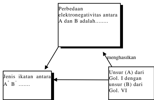
Gambar 1. Diagram Siklis Ikatan Kimia
