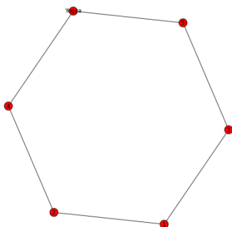
Gambar 1: Graf G dengan 6 simpul
