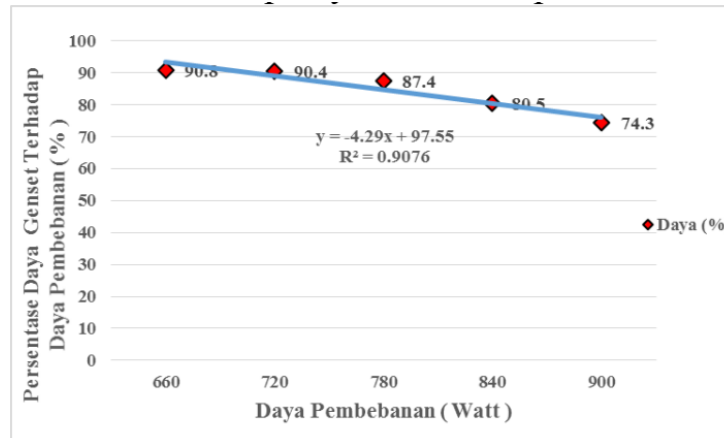
Gambar 3.3 Pengaruh daya pembebanan terhadap persentase daya genset
