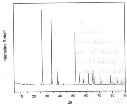
Gambar 1. Difraktogram Sinar-X SnO 2 Hasil Sintesis
