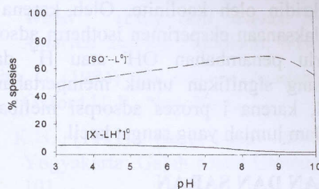
Gambar 7. Distribusi kompleks yang terbentuk pada adsorpsi 1 mM 9-aminoakridin oleh kaolinite, yang dihitung berdasarkan parameter yang tertera dalam Tabel 1.
