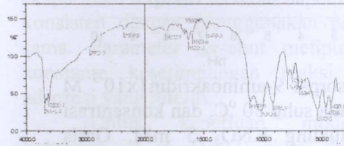
Gambar 6. Spektrogram IR kaolinite setelah adsorpsi 9-aminoakridin
