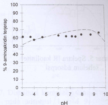
Gambar 3. Adsorpsi 9-aminoakridin 1x10 -3 M oleh kaolinit pada suhu 30 °C, dan konsentrasi elektrolit pendukung KNO 3 5 mM. Garis merupakan hasil pemodelan dengan parameter dicantumkan pada Tabel 1.
