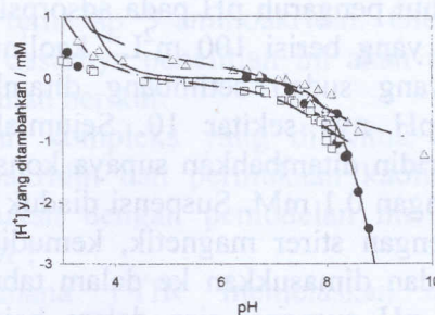
Gambar 2. Titirasi (●) 0.01M 9-aminoakridin, (□) 100 \text{ m}^2 \text{ L}^{-1} kaolinite, dan (Δ) suspensi berisi 100 \text{ m}^2 \text{ L}^{-1} kaolinite dan 0.1mM 9-aminoakridin. Garis merupakan hasil hitung dengan menggunakan parameter yang dicantumkan dalam Tabel 1.
