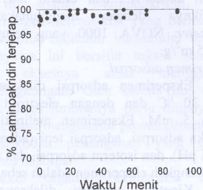
Gambar 1. Kinetika adsorpsi 0.1 mM 9-aminoakridin oleh 100 \text{ m}^2 \text{ L}^{-1} kaolinite pada suhu 30^\circ \text{C} dan pH 4.
