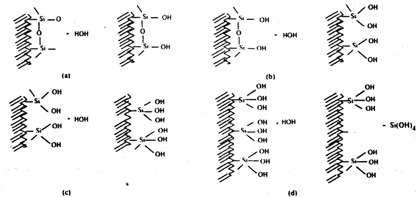
Gambar 4. Hidrolisis pada spesies permukaan silika
