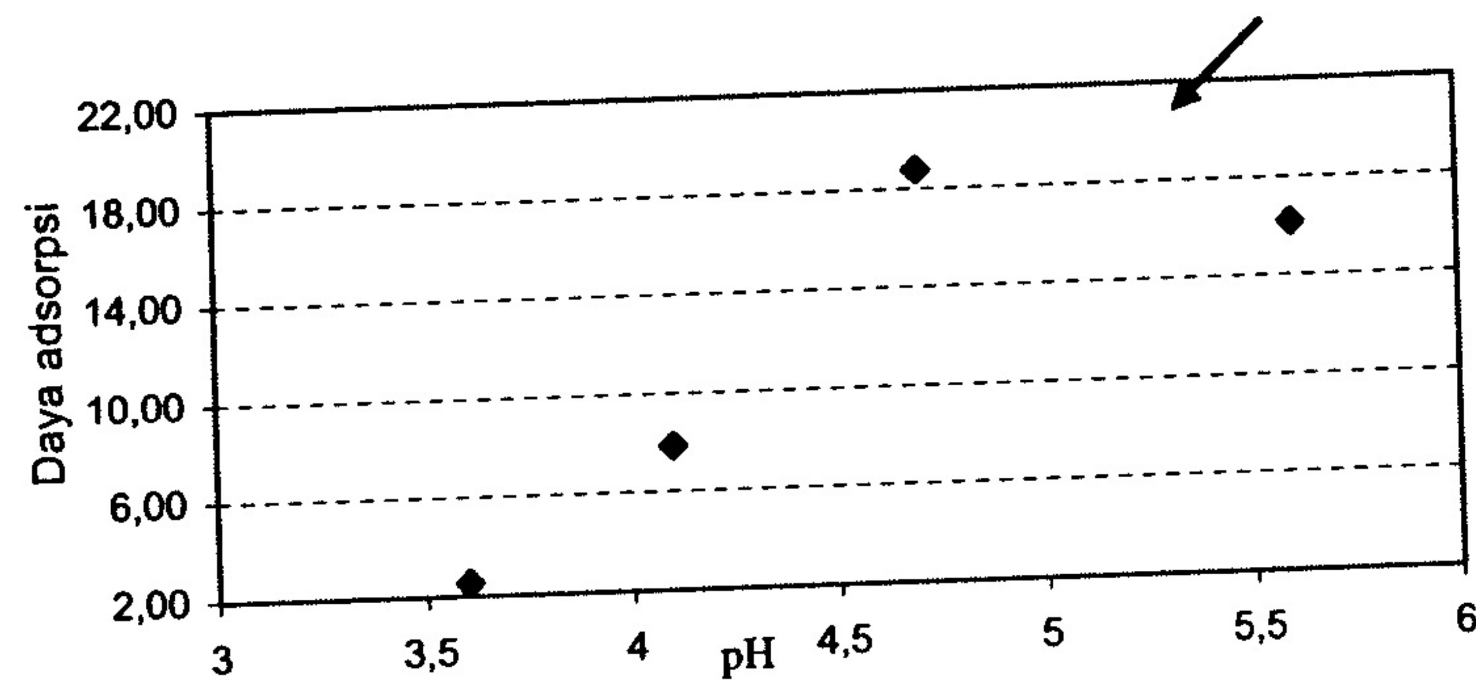
Gambar. 2. Daya adsorpsi kitosan terhadap Cr(III) pada berbagai pH sistem
