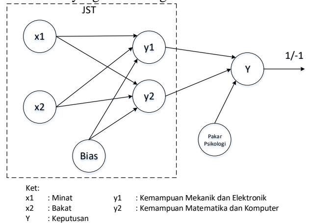
Gambar 8. Sistem JST Tes Minat dan Bakat Bidang Robotika
